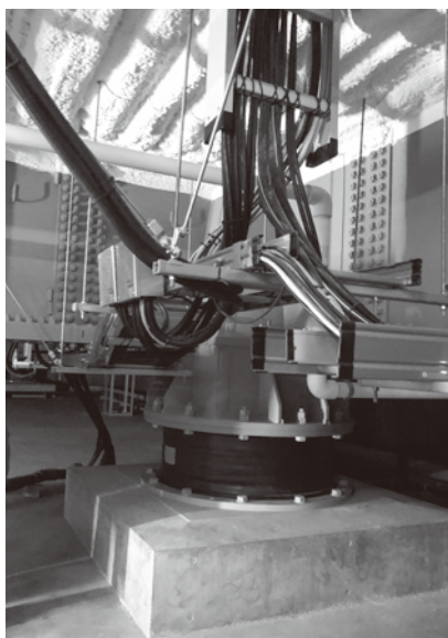
庁舎地下の免震構造
