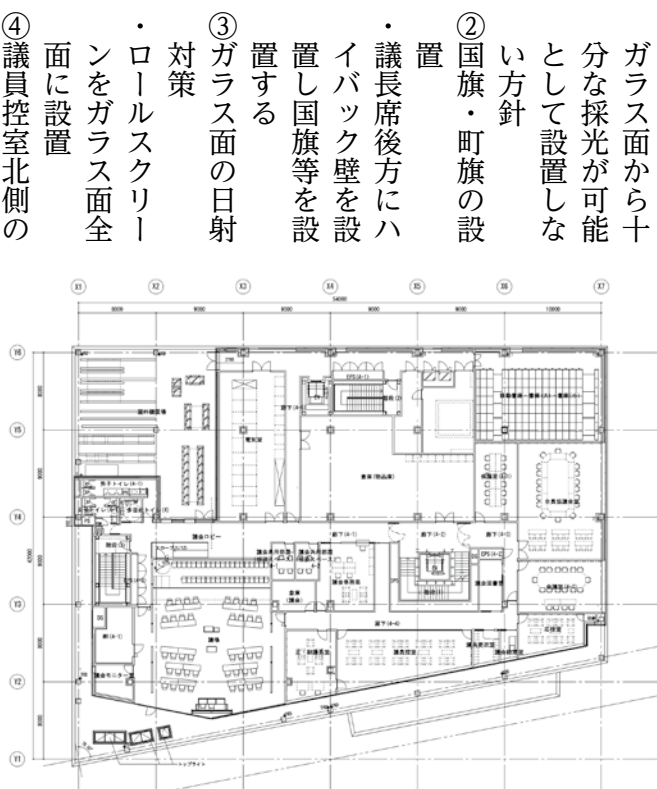
新庁舎4階議会フロアのレイアウト図(案)
